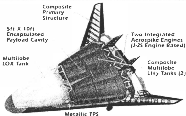
Enkel planritning över prototypfarkosten X-33. (Bild:NASA)
